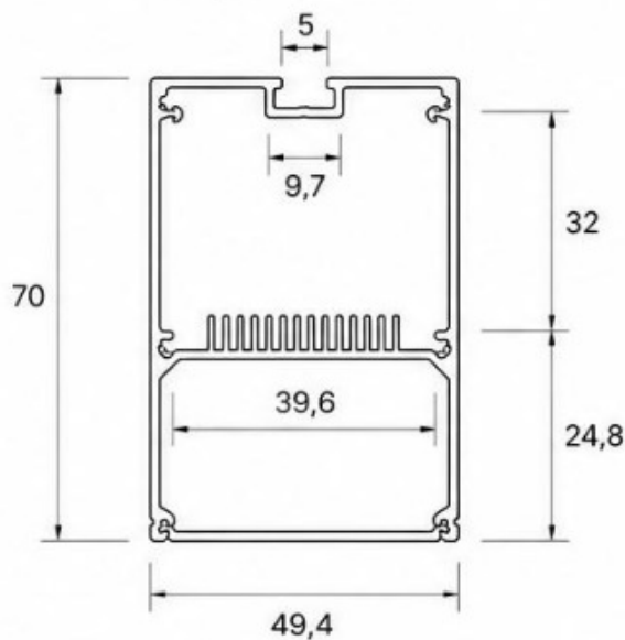
Профиль 70×49,4 мм
