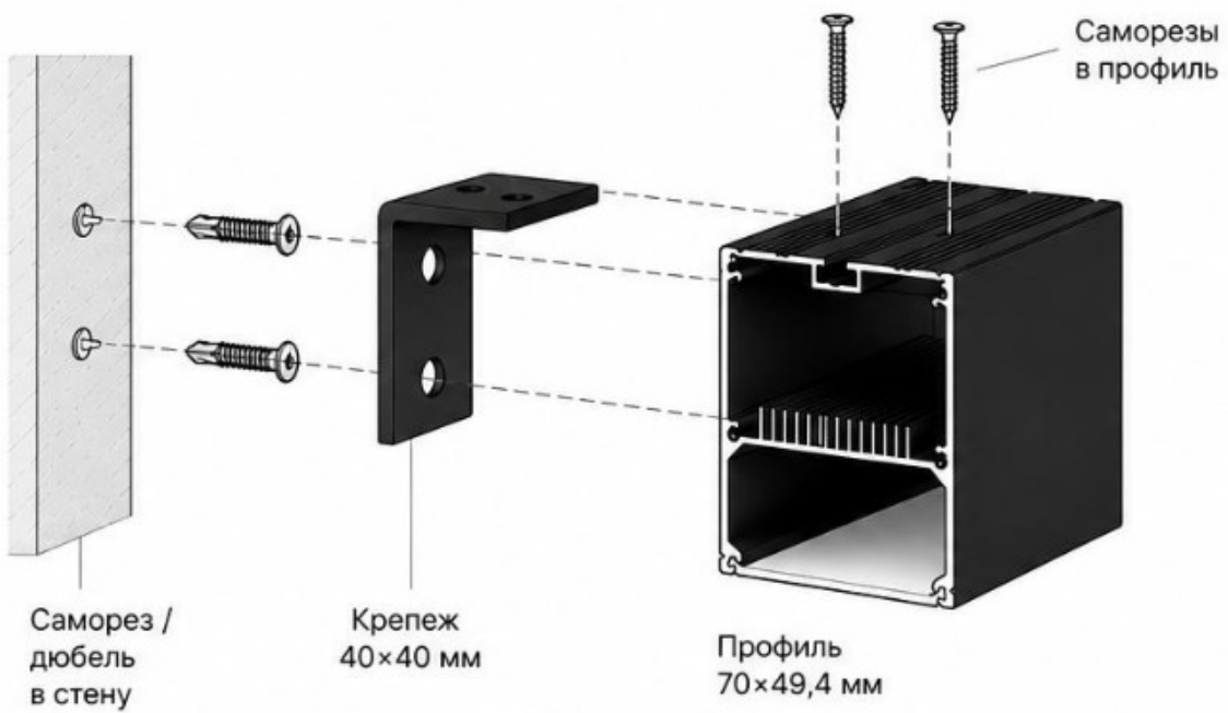
Профиль 70×49,4 мм
