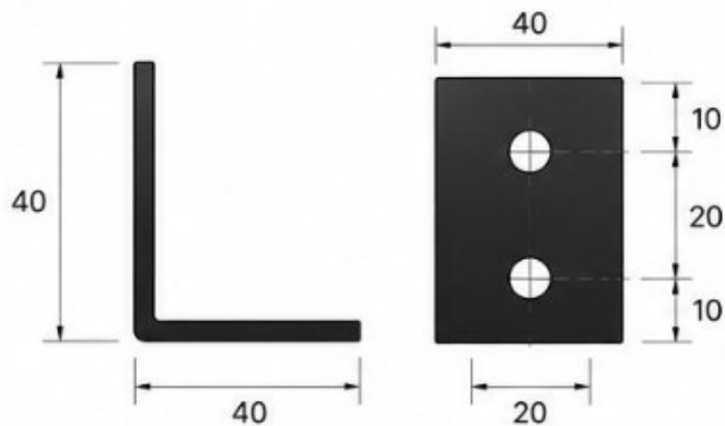
Крепеж 40×40 мм
